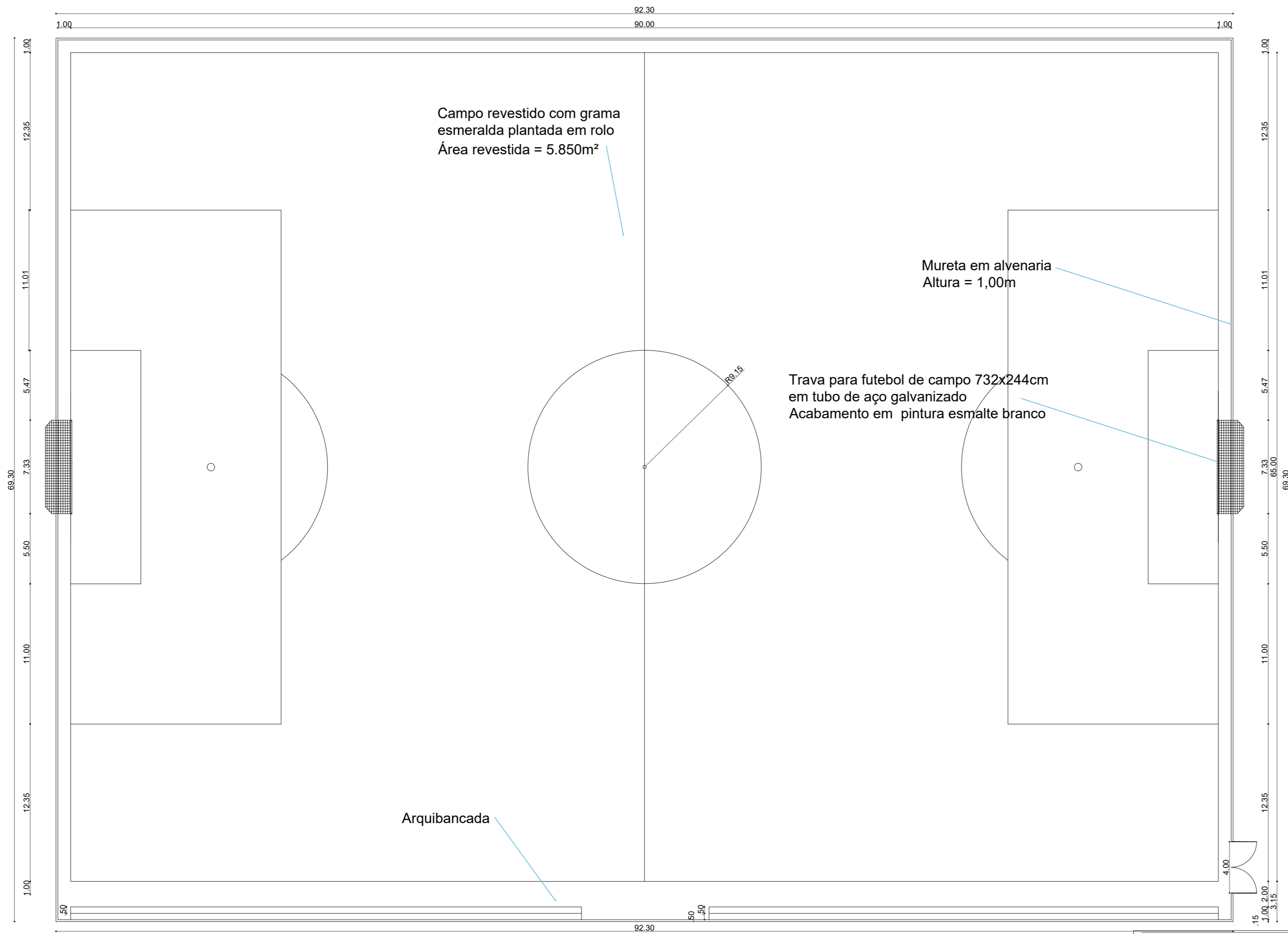
1 PLANTA BAIXA esc 1:250
