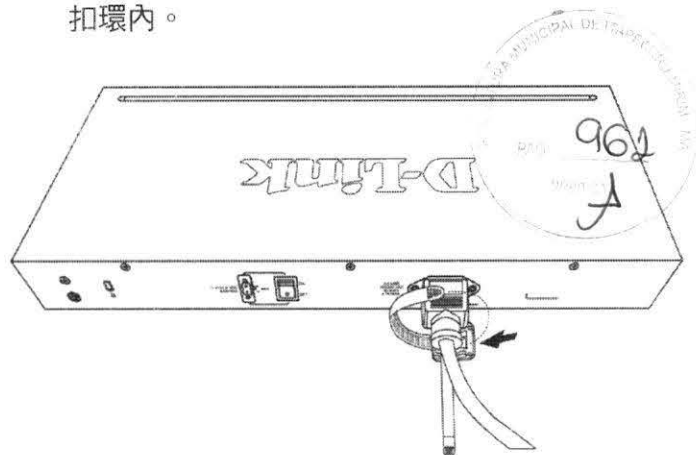
將固定器上的束帶纏繞電源線
