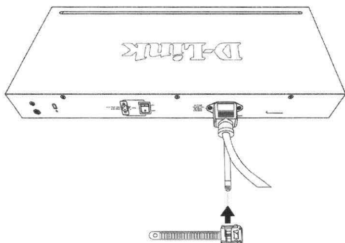
Pasang pengikat untuk tie wrap
