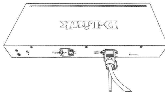
Закрепление кабеля питания
