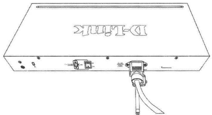
Mengamankan kabel listrik
