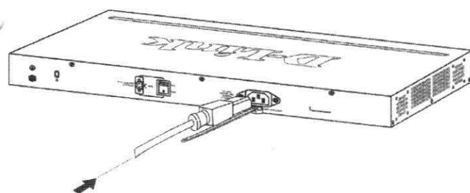
連接電源線至交換器
