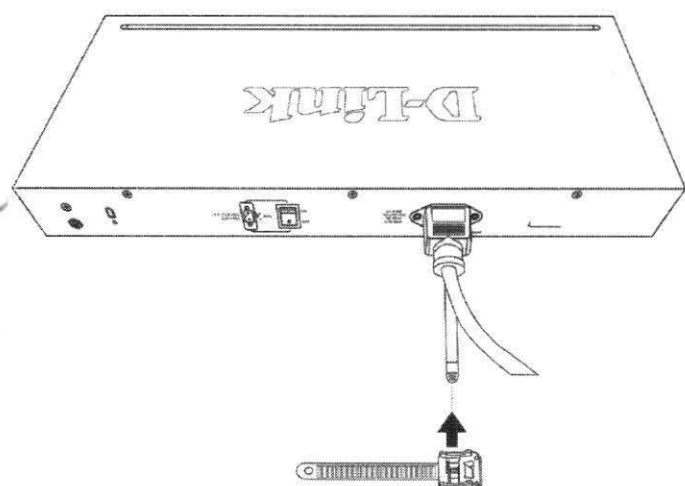
將固定器插入束帶
